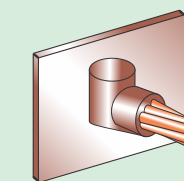
Conexão Cabo à Superfície de Aço
